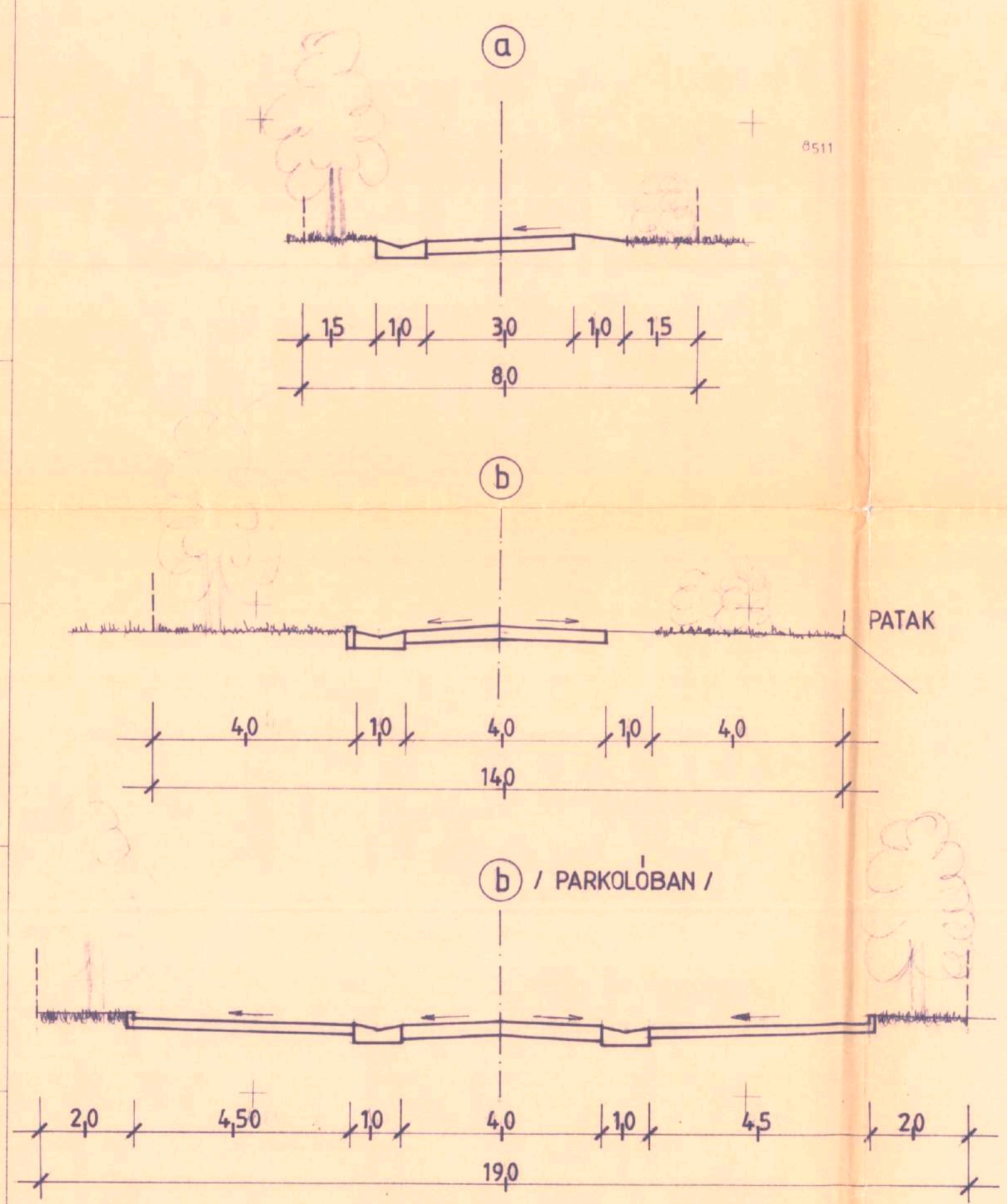
JAVASOLT ÚT-KERESZTMETSZETEK M=1:100
